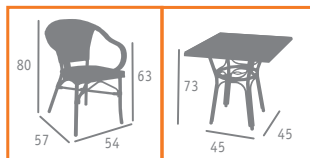
▶▶ SILLÓN MOD. MANILA PINTADO DECO - NOGAL (Ø 28) TEXTILENE ROJO
