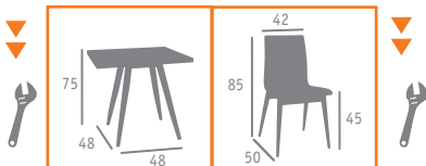
▲ SILLA MOD. MÍCHIGAN C4 ACERO PINTADO DECO MADERA NATURAL CARCASA MADERA COLOR NOGAL VINTAGE
